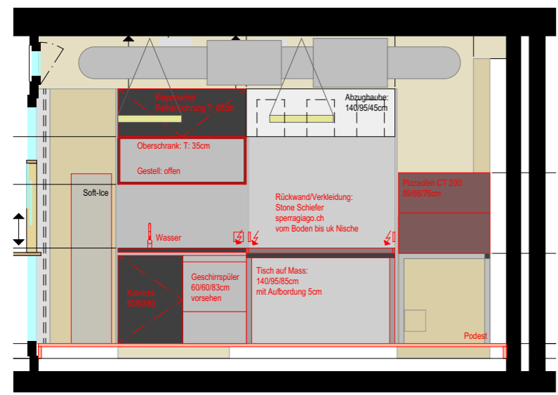
ANSICHT | Mst.: 1:50
