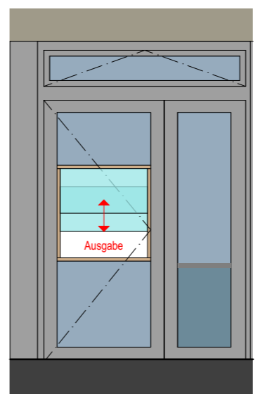
ANSICHT | Mst.: 1:50
